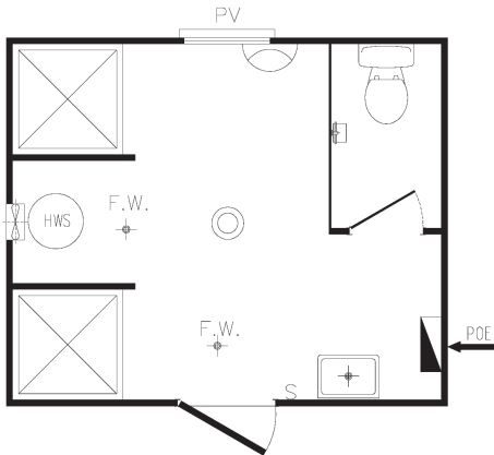
A-003 4.8 x 3.0m
