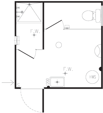
A-002 3.6 x 3.0m
