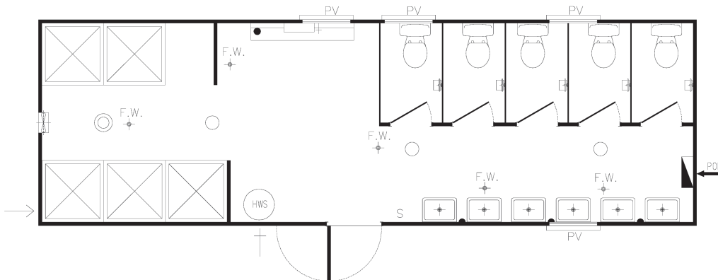
A-006 9.6 x 3.0m
