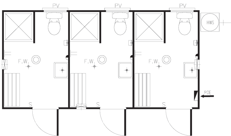
A-008 6.0 x 3.0m
