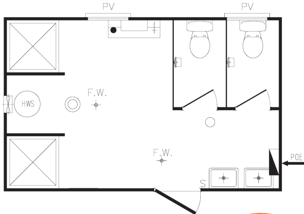
A-003 4.8 x 3.0m
